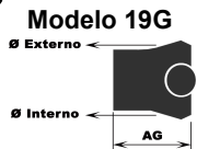
Gaxeta Modelo 19G - Indicada para Hastes e Êmbolos
